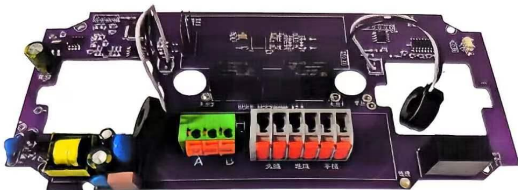
电瓶车主控板
