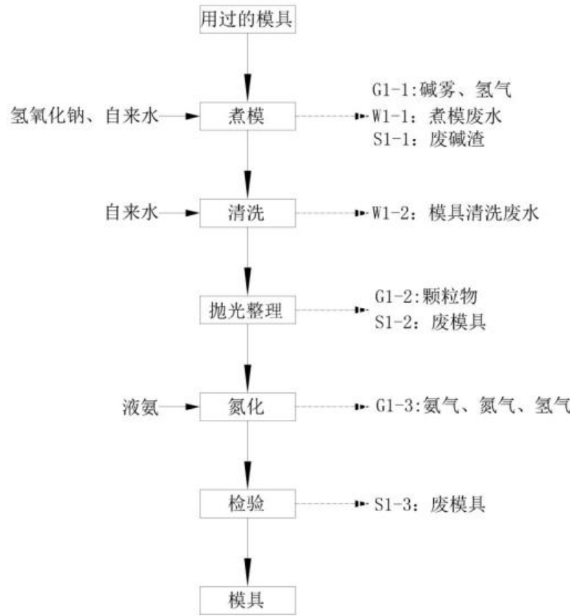
图 2.3-1 模具氮化生产工艺流程图示意图
