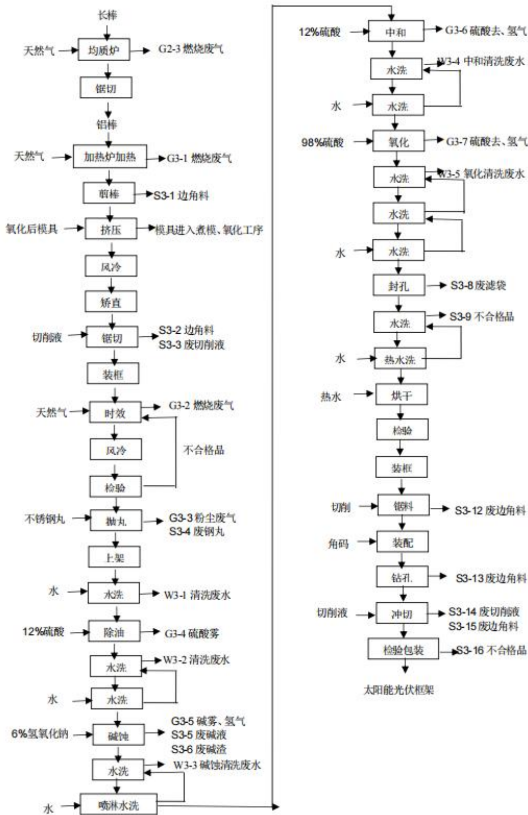
图 2.3-3 太阳能光伏框架工艺流程图
