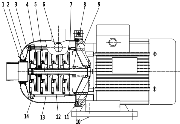
截面图 LQDWF10,12,15,20
