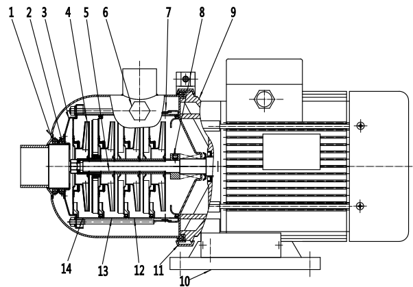
截面图 LQDWF,LQDWJ(T)
