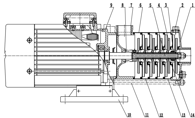
截面图 LQDWF,LQDWJ(T)
