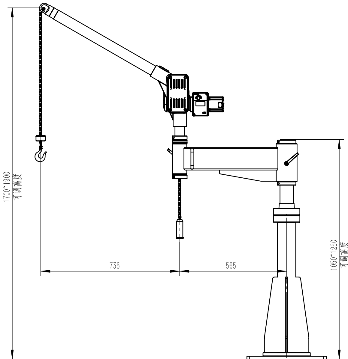
WD8900交链式微吊尺寸
