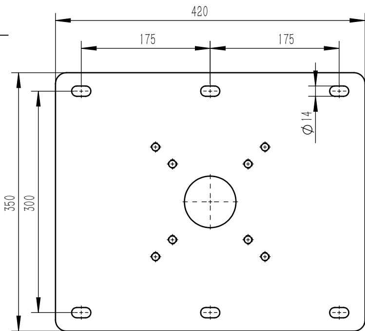
固定底板尺寸
