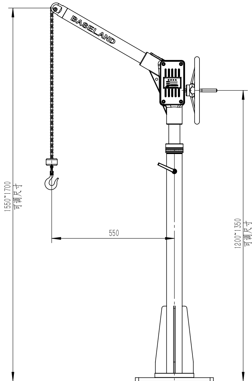
WD6000单臂吊
