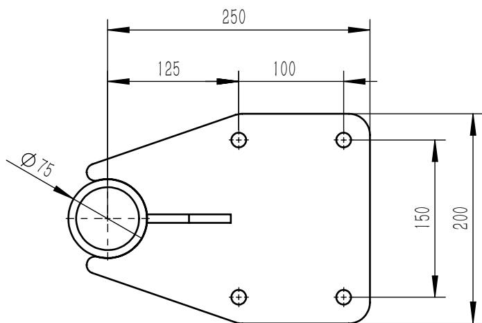
WD5000桌面单臂吊固定板
