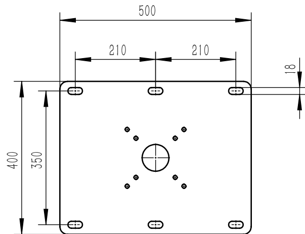
固定底板安装尺寸
