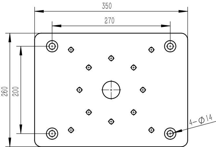
固定底板尺寸
