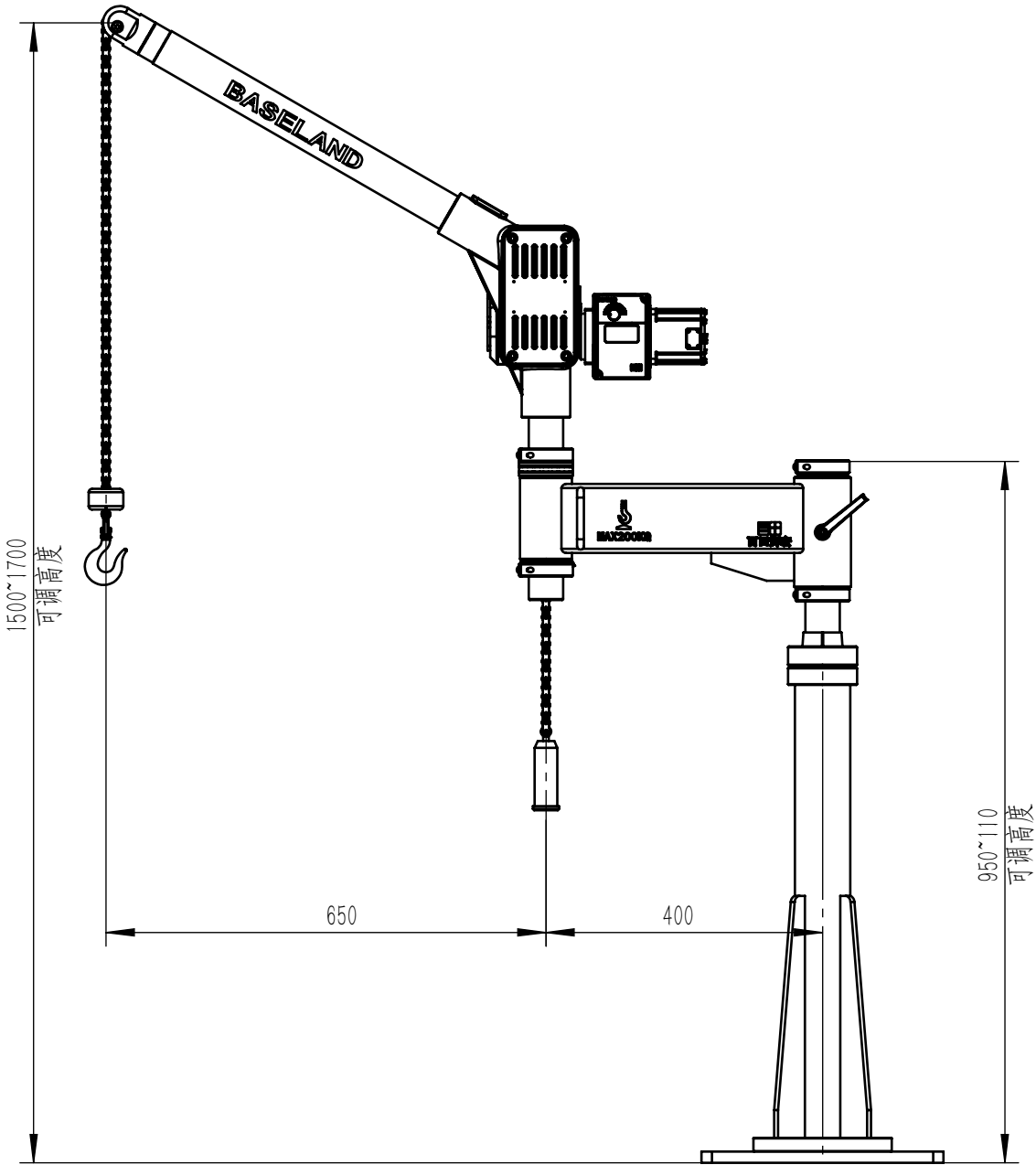
WD8800D交链式微型吊参数
