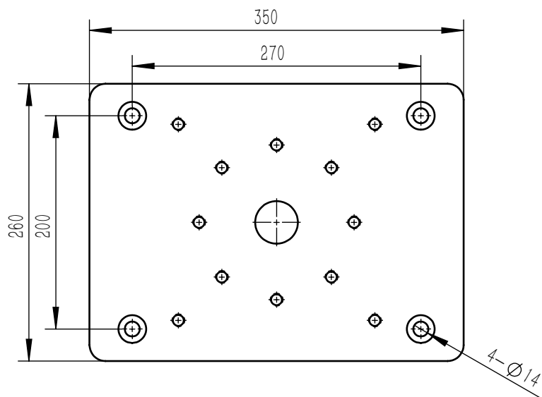
固定底板尺寸
