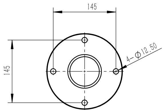
微吊底板尺寸
