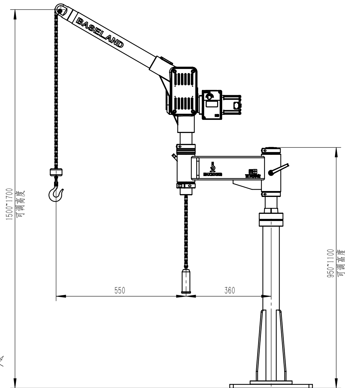
WD8700D交链式微型吊参数
