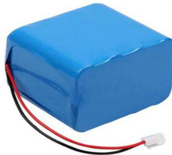
产品型号:JS-14.8V-6.6AH 尺 寸:260*55.5*23±0.5(mm)
