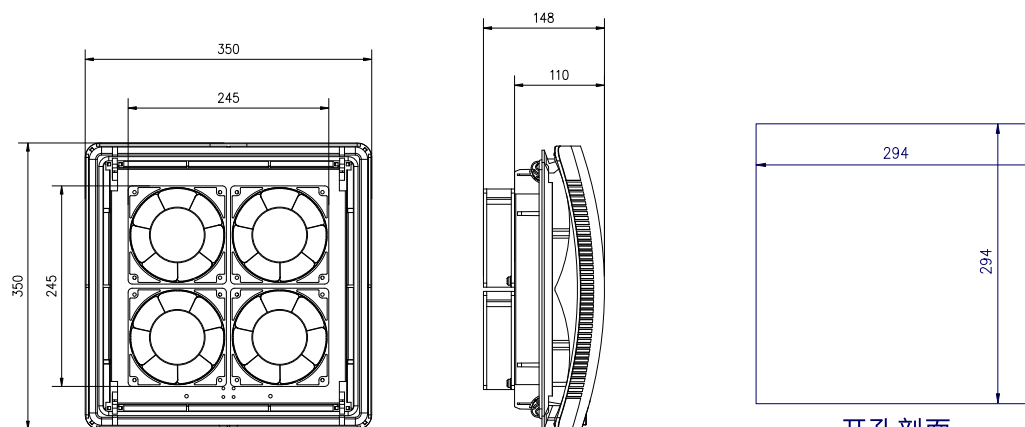
开孔剖面 OPENING PROFILE
