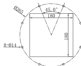
开孔剖面 OPENING PROFILE
