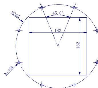
开孔剖面 OPENING PROFILE
