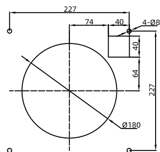
开孔剖面 OPENING PROFILE
