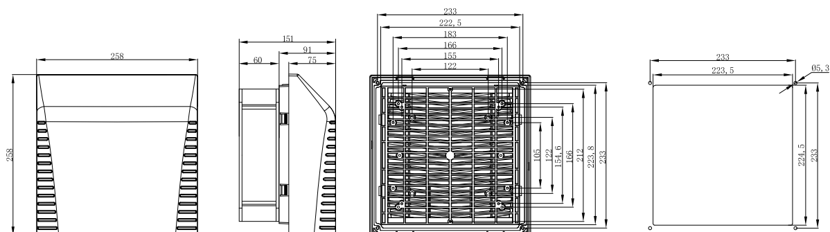
开孔剖面 OPENING PROFILE
