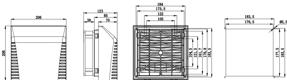
开孔剖面 OPENING PROFILE
