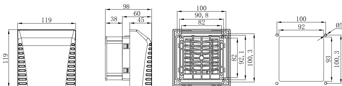
开孔剖面 OPENING PROFILE
