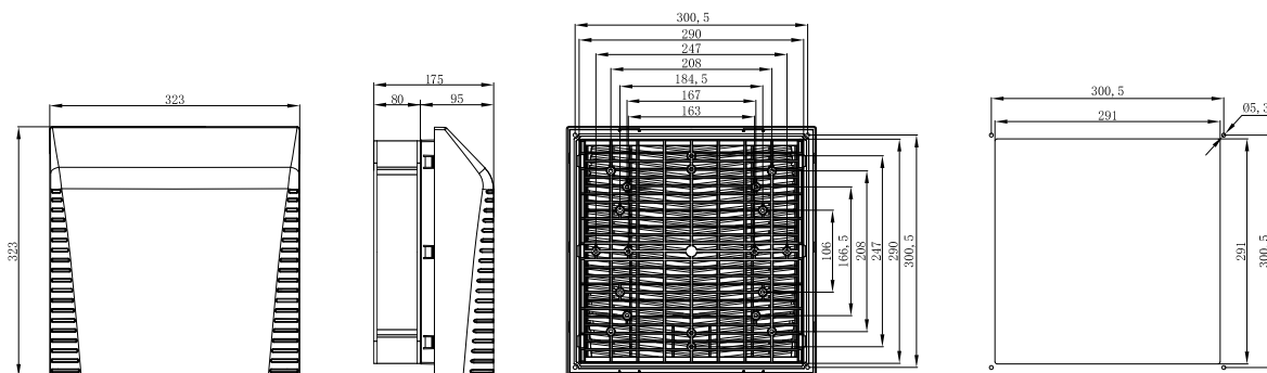
开孔剖面 OPENING PROFILE
