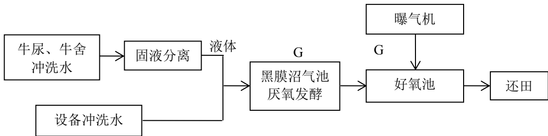
图3-4 项目运营期污水处理工艺流程图及产污节点图
