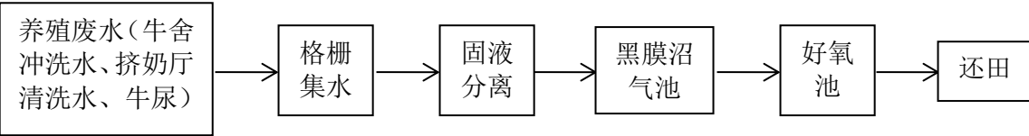
图4-1 污水处理工艺流程图
