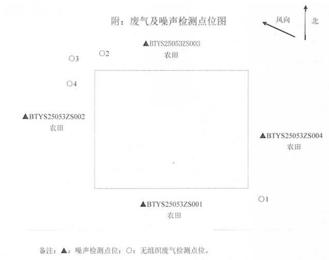
图7-1 东厂区无组织废气、噪声监测点位示意图
