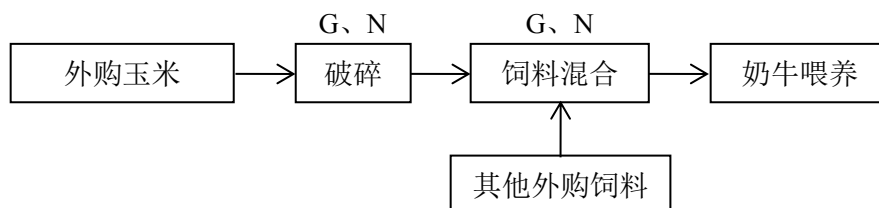
图 3-3 项目运营期饲料加工工艺流程图及产污节点图
