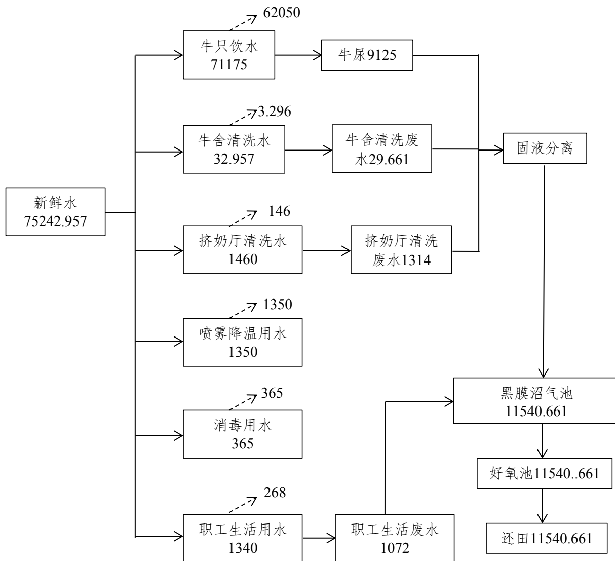
图3-1 水平衡图 (m³/a)
