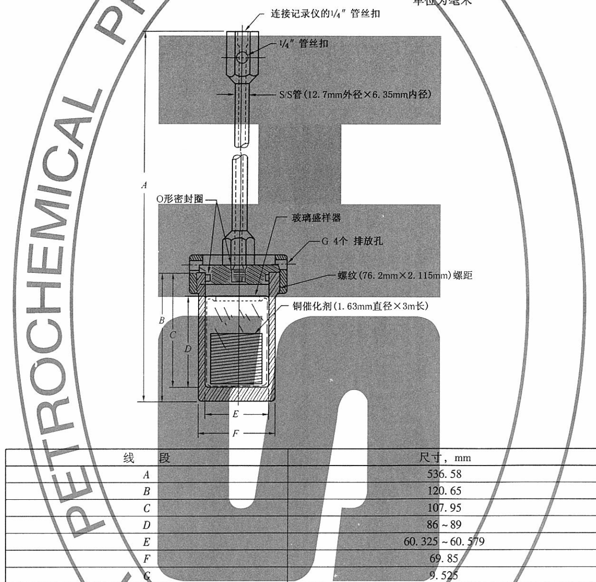
图 A.1 氧弹
