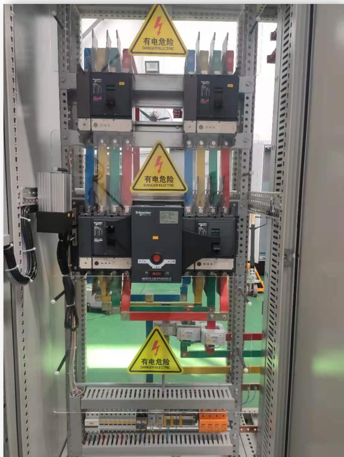
低压配电柜
